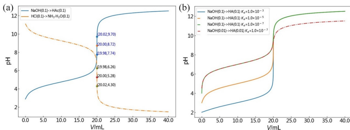
图3 \text{HAc} 和 \text{NH}_3 \cdot \text{H}_2\text{O} 的滴定曲线(a)及不同强度一元弱酸 \text{HA} 的的滴定曲线(b)
